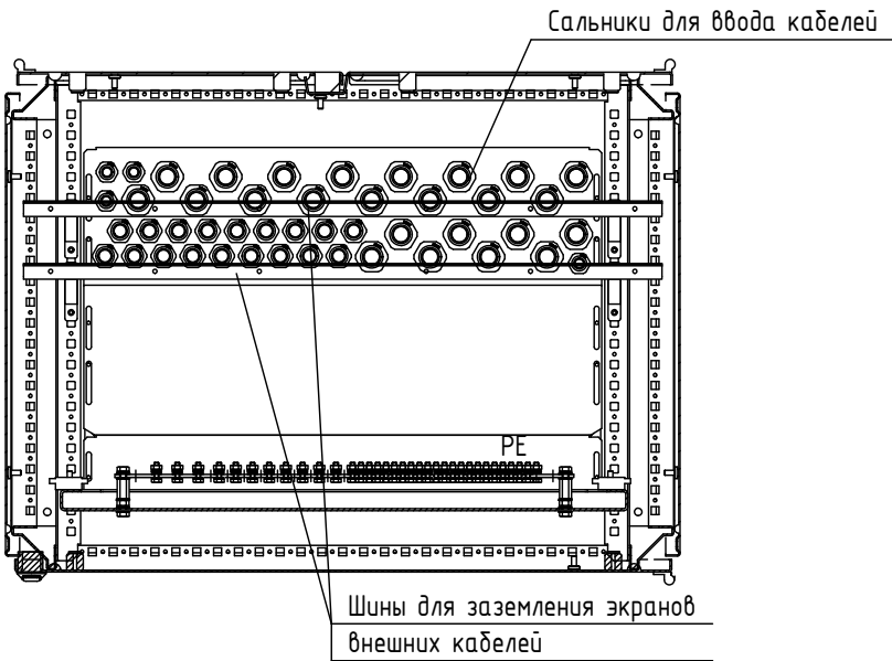
Б-Б
